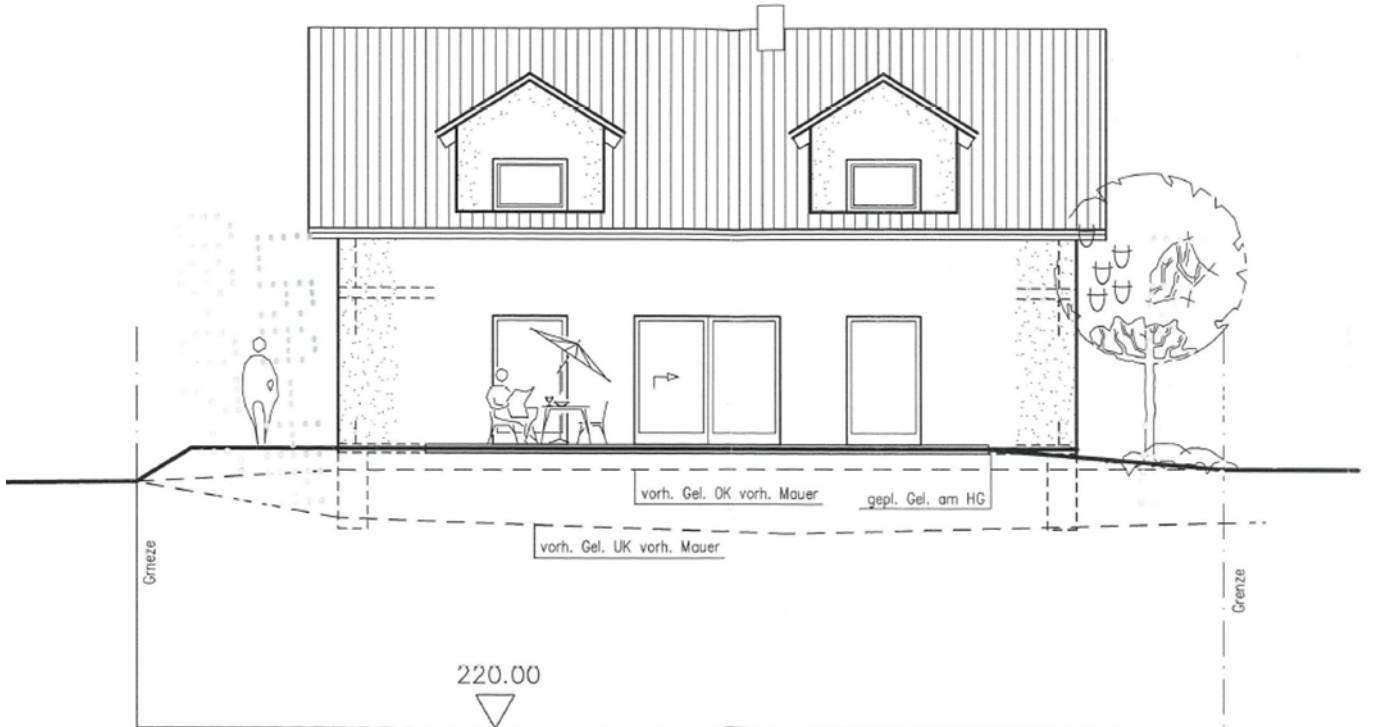
Ansicht Süd
